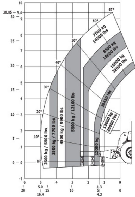
Máquina sobre neumáticos con brazo
